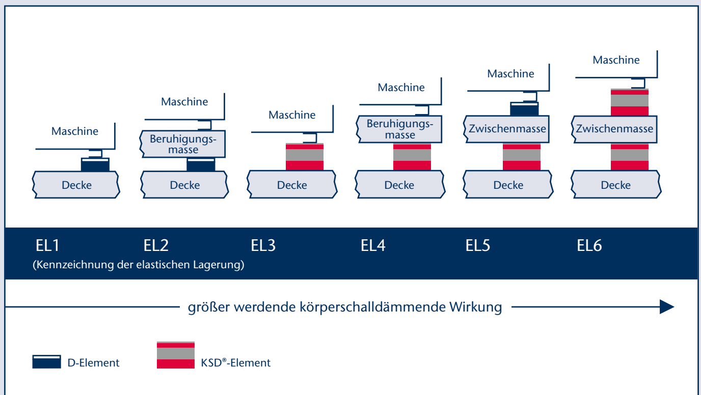
Bild 1 – Schematische Darstellung der elastischen Lagerung von Maschinen und Geräten
